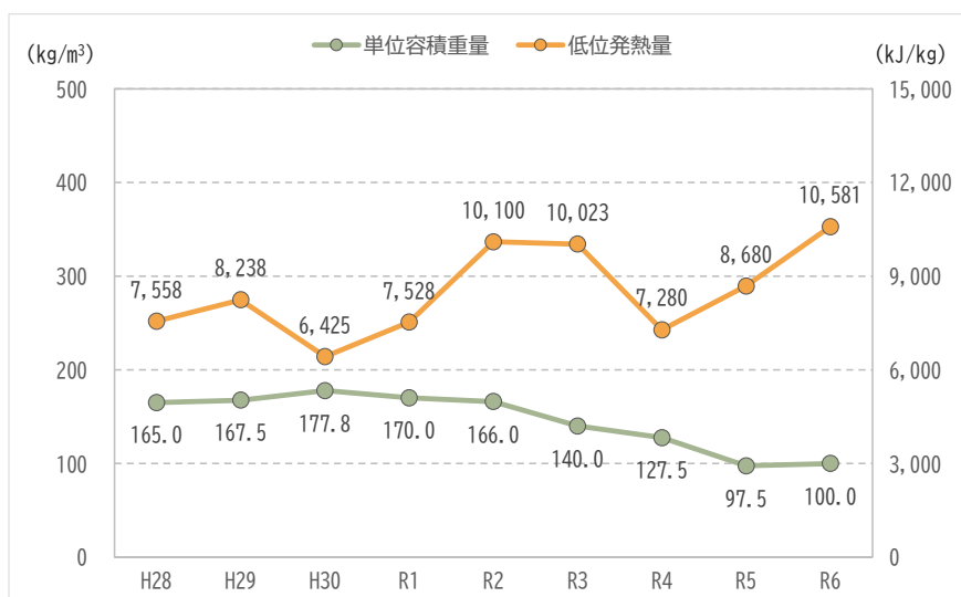
図 3.6 単位容積重量及び低位発熱量の推移 (いなべ市)
