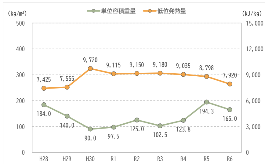
図 3.8 単位容積重量及び低位発熱量の推移（菰野町）
